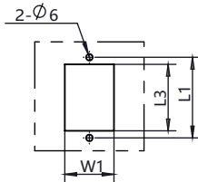
面板安装尺寸
