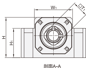
剖面A-A
