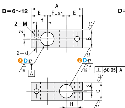
同径直交反向型
