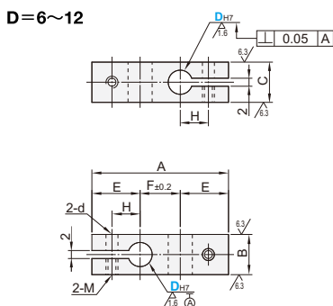
同径直交反向型
