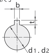
键槽尺寸
