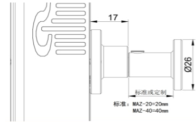
MAZ-20 MAZ-40 -背面解锁组件尺寸图
