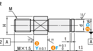
螺纹长度固定型
