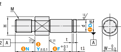
螺纹长度指定型
