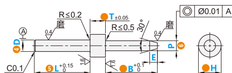
锥头型 DAVZKR DAVZS
