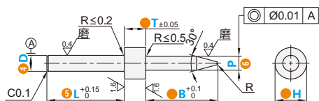
锥头R型 DAVJKR DAVJS
