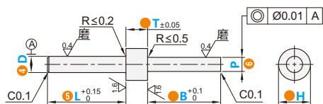
平头型 DAVGKR DAVGS
