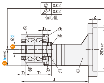
剖面B-B
