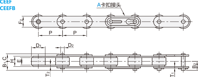
双节距大滚子输送链条
