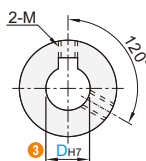
安装方式 (键槽+螺孔) N
