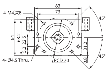
B向
