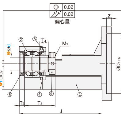
剖面B-B
