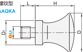
外螺纹型 GAAQKB
