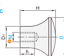
内螺纹型 GAAQKC
