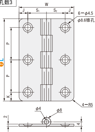
单侧孔数3
