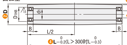
圆弧型
