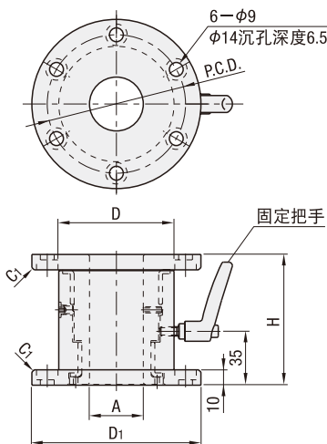
双侧法兰 (HRCNW)
