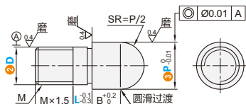
大头外螺纹型 DAXCS DAXCSSR
