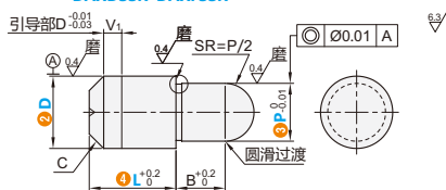
小头内螺纹型 DAXGS DAXGSSR
