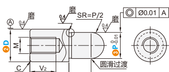
小头内螺纹型 DAXGS DAXGSSR
