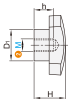
内螺纹型 GAAUKK(M5A/M6A/M8A/M10A)
