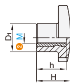
内螺纹型 GAAUKK(M4/M5/M6/M8)
