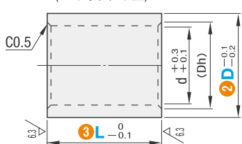
(L尺寸负公差)
