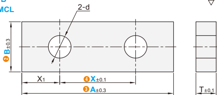
通孔型-双孔型 ECBLPB ECBMMCL
