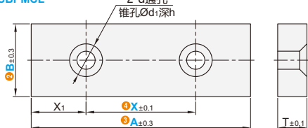
锥孔型 ECBNPB ECBPMCL
