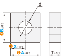
通孔型-单孔型 ECBJPB ECBKMCL
