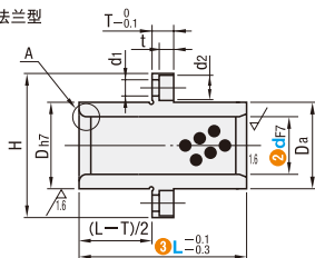
中间法兰型
