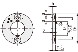
AFWZ (平头螺栓型)
