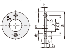
AFWTZ (短头螺栓型)
