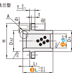
圆法兰型
