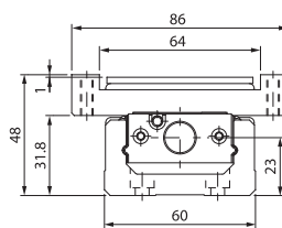
剖面: A-A
