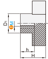
内螺纹型 GAARKG
