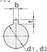
键槽尺寸
