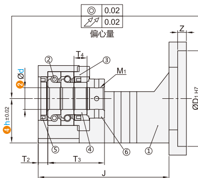
剖面B-B
