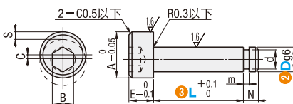
DBJP (挡圈型)
