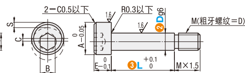
DBJPB (螺帽固定型)
