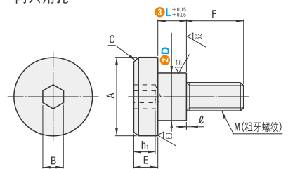
内六角孔
