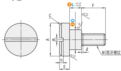
一字槽
