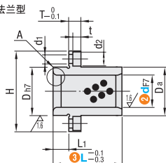
嵌入式法兰型
