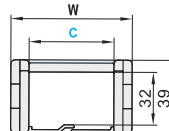
内径开口 AHZ16
