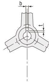
轴孔键槽详图
