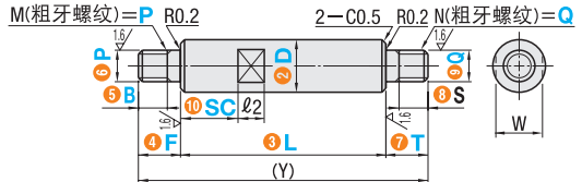
带扳手槽型
