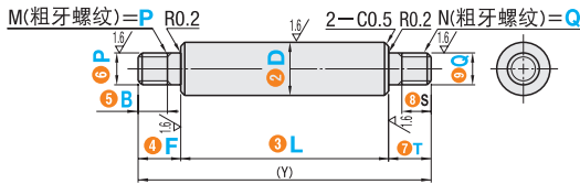
①D部公差h9/P·Q部公差h7 ②D部公差h9/P·Q部公差g6型
