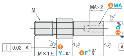
螺纹长度固定型
