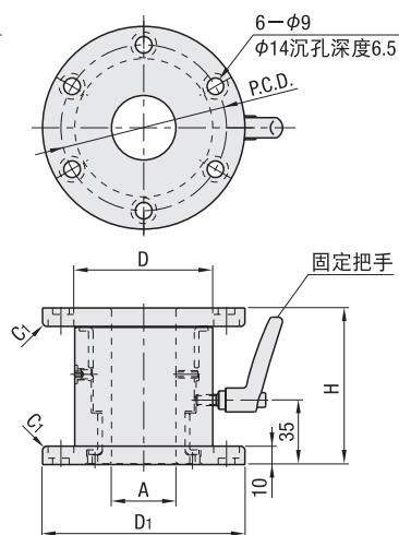
双侧法兰 (HRCNW)
