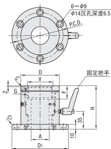
单侧法兰 (HRCN)
