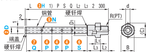
外螺纹型
