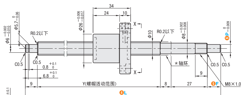
* 附属轴环(1个) 材 质 S45C 表面处理 发黑
