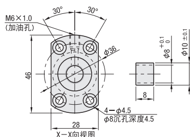
* 附属轴环(1个) 材 质 S45C 表面处理 发黑
