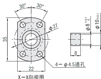
* 附属轴环(1个) 材 质 S45C 表面处理 发黑
