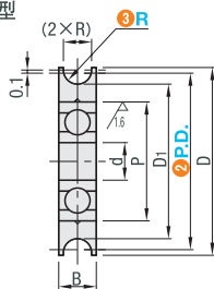
外螺纹型
