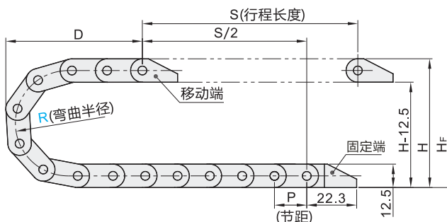
外径开口
