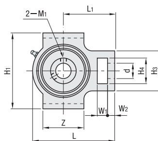
BADTKP (张紧型)
