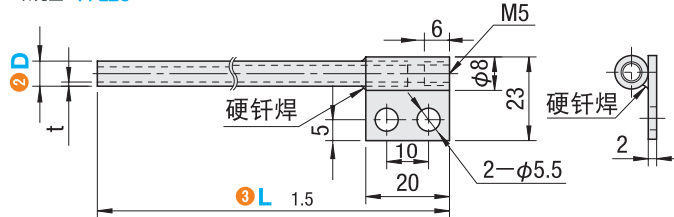
双孔型: FFLZC
