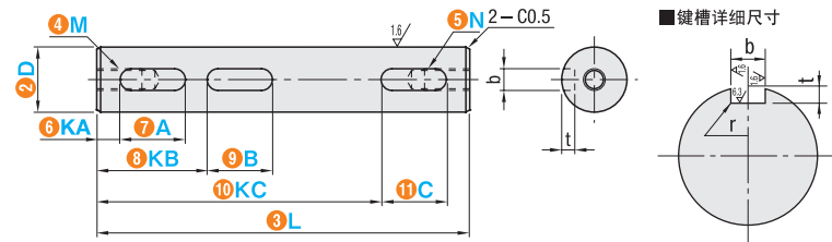
■ 键槽详细尺寸
