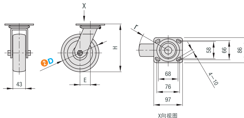
X向视图
