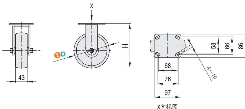
X向视图
