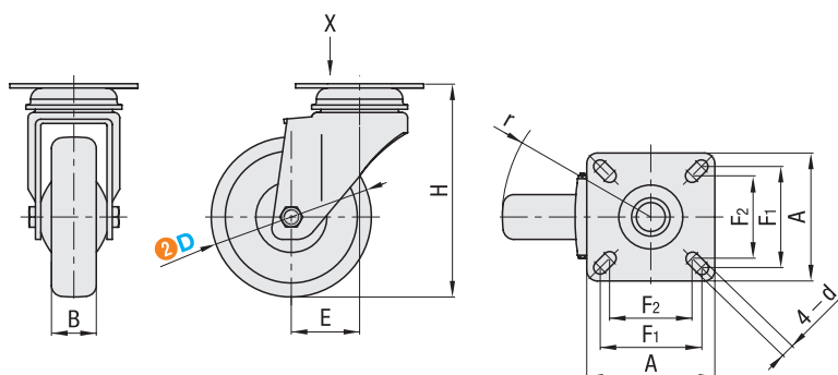
X向视图
