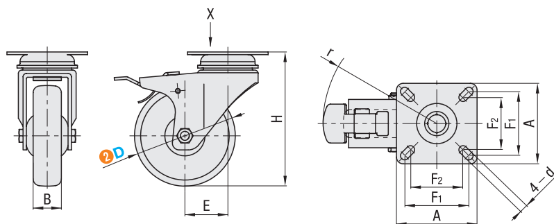
X向视图
