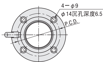
圆法兰型
