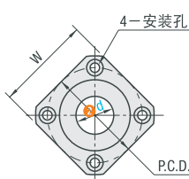
方法兰型
