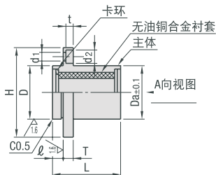
圆法兰型
