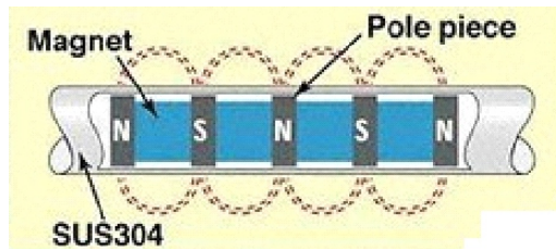
内部结构图
