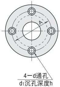
4点固定
