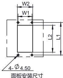
面板安装尺寸
