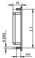
面板安装尺寸
