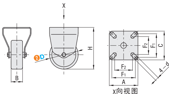
X向视图
