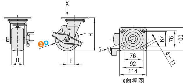
X向视图
