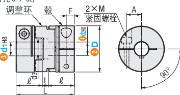
CAOCLK (带键槽孔 d1) CAOCRK (带键槽孔 d2) CAOCWK (带键槽孔 d1、d2)
