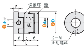
CAOLK (带键槽孔 d1) CAORK (带键槽孔 d2) CAOWK (带键槽孔 d1、d2)
