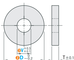
垫圈
