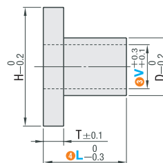
肩型轴环
